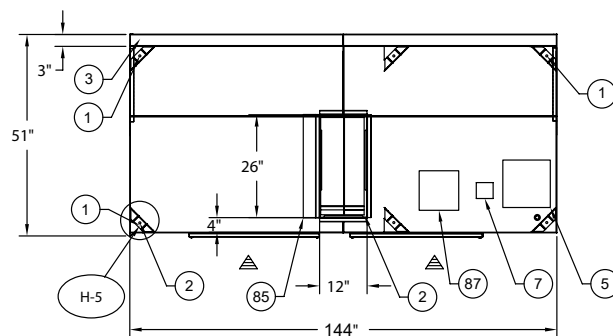
STADIUM ST-40-T VUE DE HAUT
