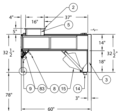
STADIUM ST-20-T VUE DE COTÉ
