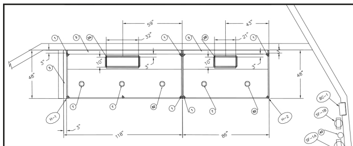
PLAN D'UNE HOTTE
