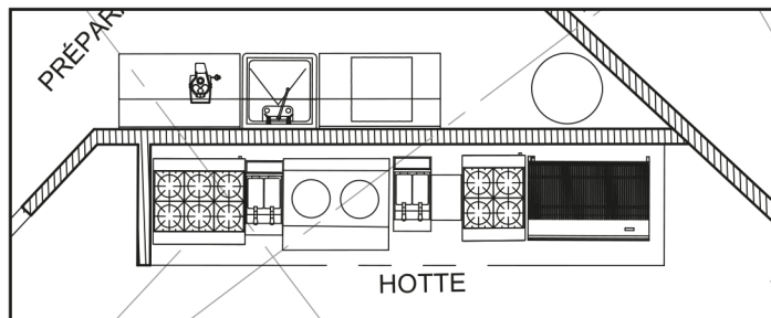
PLAN DES ÉQUIPEMENTS DE CUISSON
