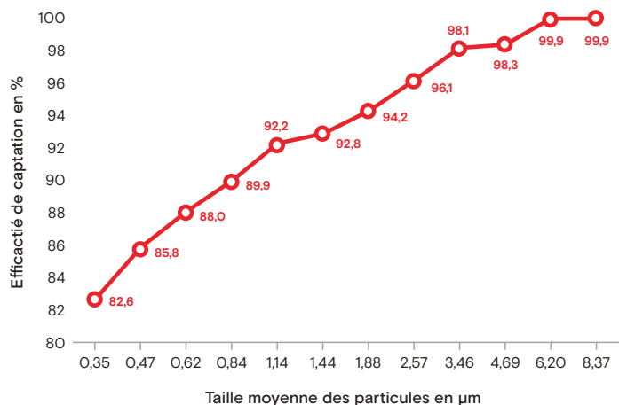
Efficacité de captation vs taille des particules selon les standard ASHRAE 52.2 (unité double passe)
